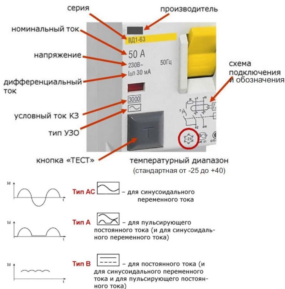
Рисунок 5. Маркировка УДТ
