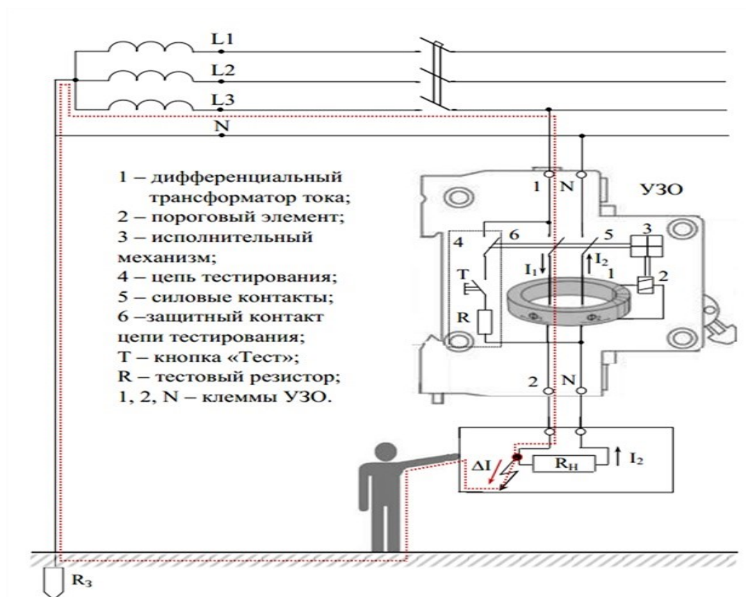
Рисунок 3. Принцип работы УДТ
